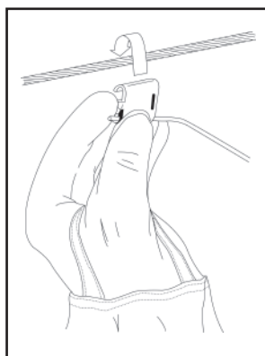
1- Coloque o condutor derivação no canal inferior do componente "C".
