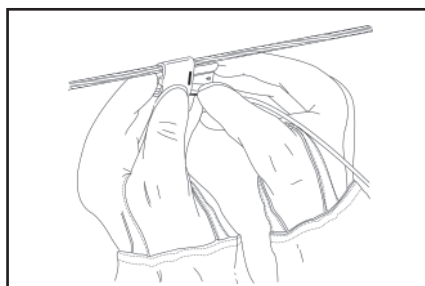
3- Ajuste e fixe o componente "cunha" entre os condutores usando apenas a pressão dos dedos, verificando a posição correta da trava.
