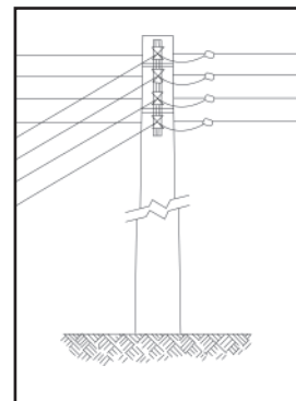
Ramal de baixada em secundário de cobre
