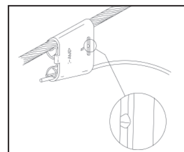
5- Certifique-se que a aplicação está correta, verificando se a trava do componente "cunha" está inserida na janela do componente "C".
