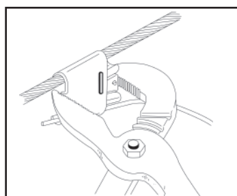
4- Complete a conexão usando o alicate tipo Bomba D'água de 12" para todos os tipos de conectores. Largura máxima do alicate na garra: 8,5mm.
