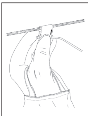
2- Acomode o componente "C" juntamente com a derivação no condutor principal mantendo o conjunto fixo com a mão.
