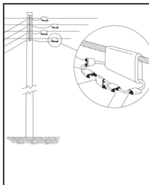
Ramal de baixada em secundário de alumínio usando "Estribo"
