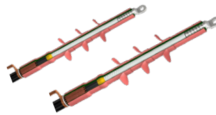
WARMSCHRUMPFENDVERSCHLÜSSE BIS 123 kV (IEC)
