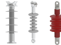
SILIKON- UND EVA-ISOLATOREN BIS 72 kV
