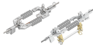
REIHENTRENSCHALTER UND SICHERUNG FÜR FLIEGENDE MONTAGE
