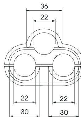
Kabelzugang
