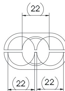
Kabelzugang
