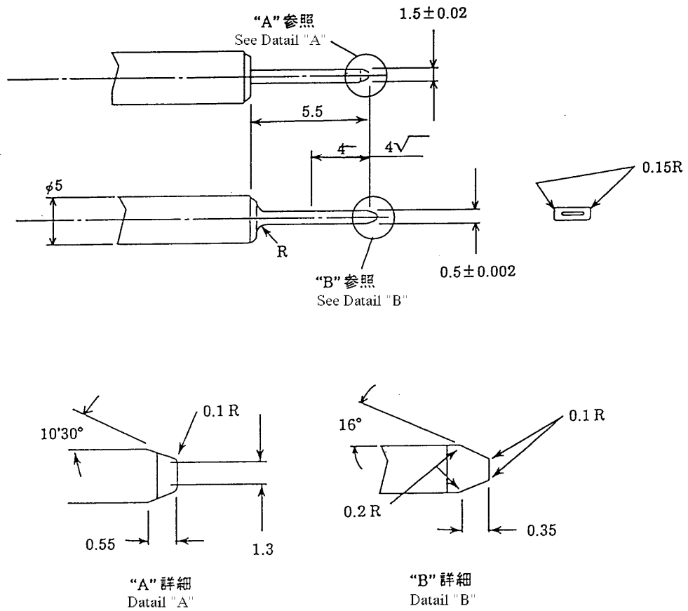
Fig. 7 コンタクト挿入引抜き力測定用ゲージ
